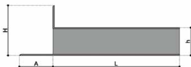
MAPEPLAN T NÉGYSZÖGLETES VÍZKÖPŐ
