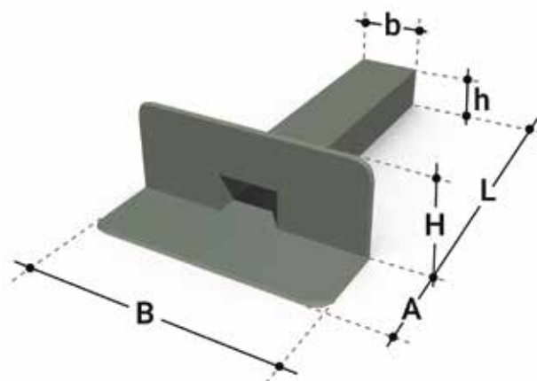
MAPEPLAN T NÉGYSZÖGLETES VÍZKÖPŐ
