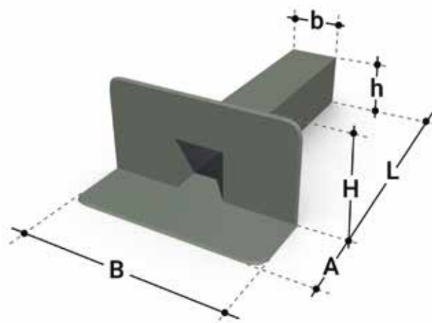
MAPEPLAN T NÉGYZETES VÍZKÖPŐ
