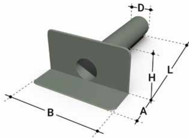
MAPEPLAN T KÖRALAKÚ VÍZKÖPŐ
